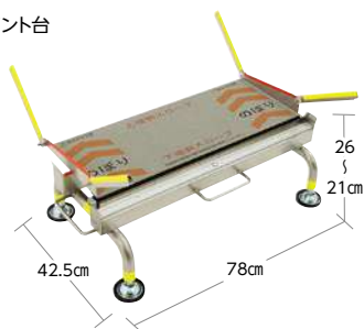
ジョイント台
