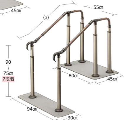
階段タイプ 両側手すり
